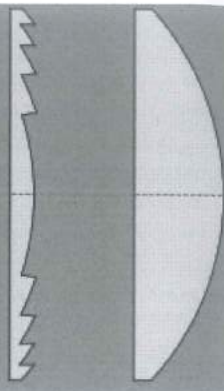
Abb. 3: Fresnel-Linse
